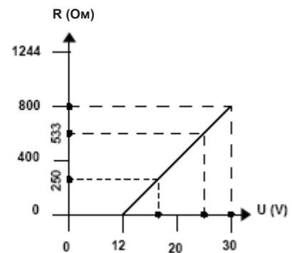
Rosemount 3107 и Rosemount 3108
